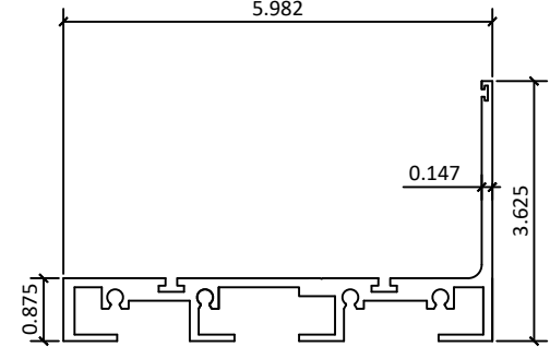
2 2800-03 – SILL
