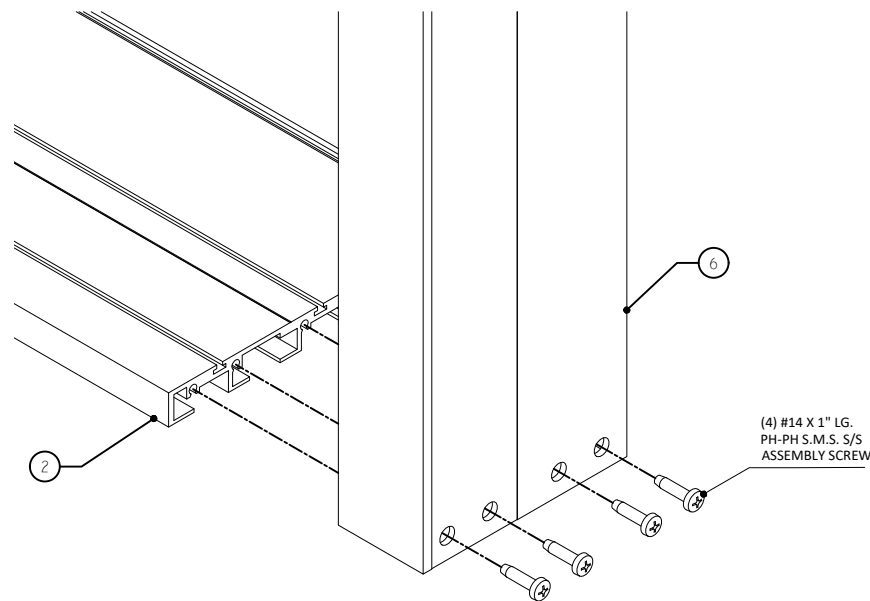
DOOR FRAME BOTTOM CORNER
