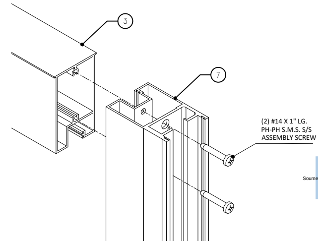
DOOR PANEL TOP CORNER
