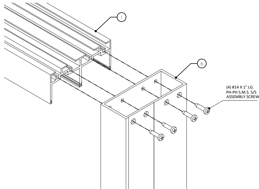
DOOR FRAME TOP CORNER
