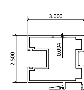
10 2800-11 – INTERLOCK
