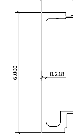
9 2800-22 – JAMB FIXED
