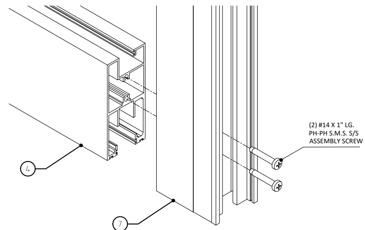
DOOR PANEL BOTTOM CORNER
