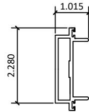
19 2800-06 - ASTRAGAL
