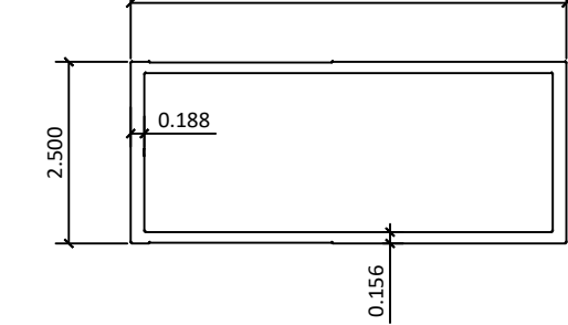
6 2800-04 – JAMB
